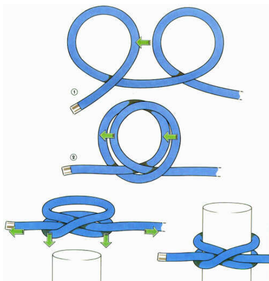
Mastwurf gelegt
