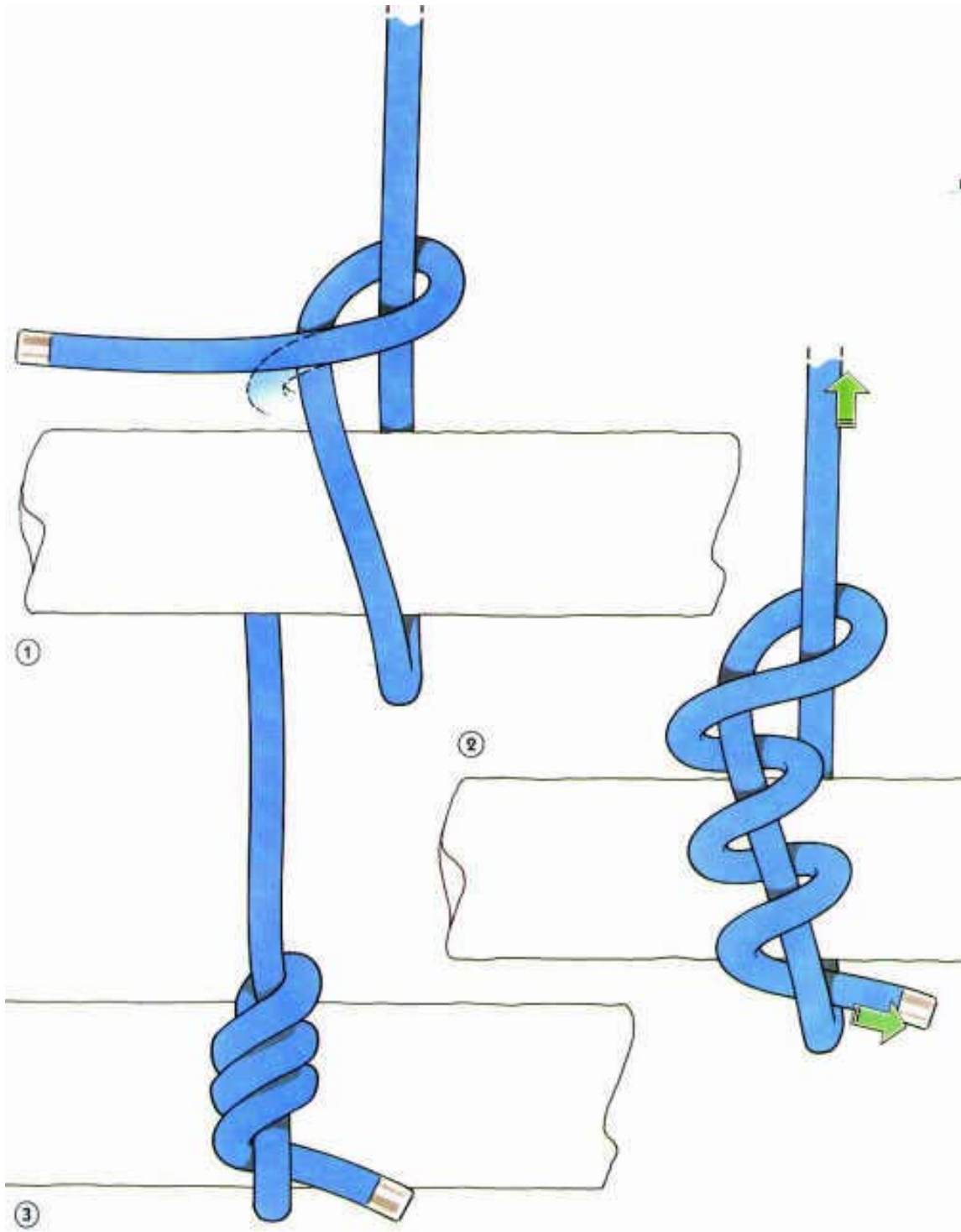
Zimmermannsschlag
