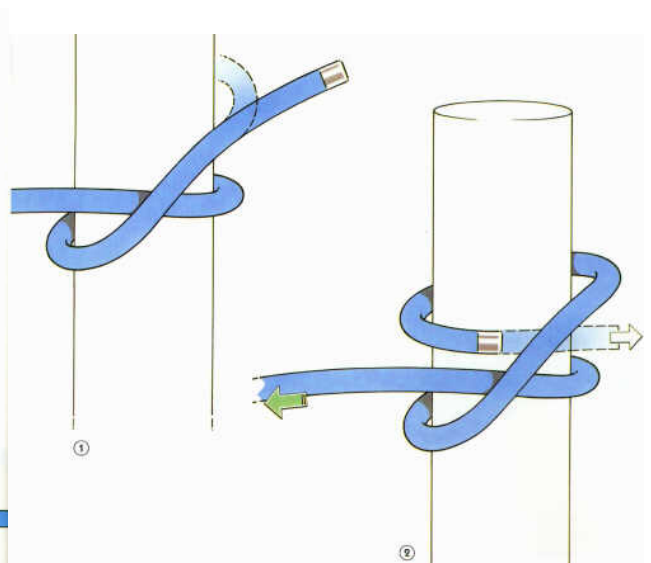
Mastwurf gesteckt
